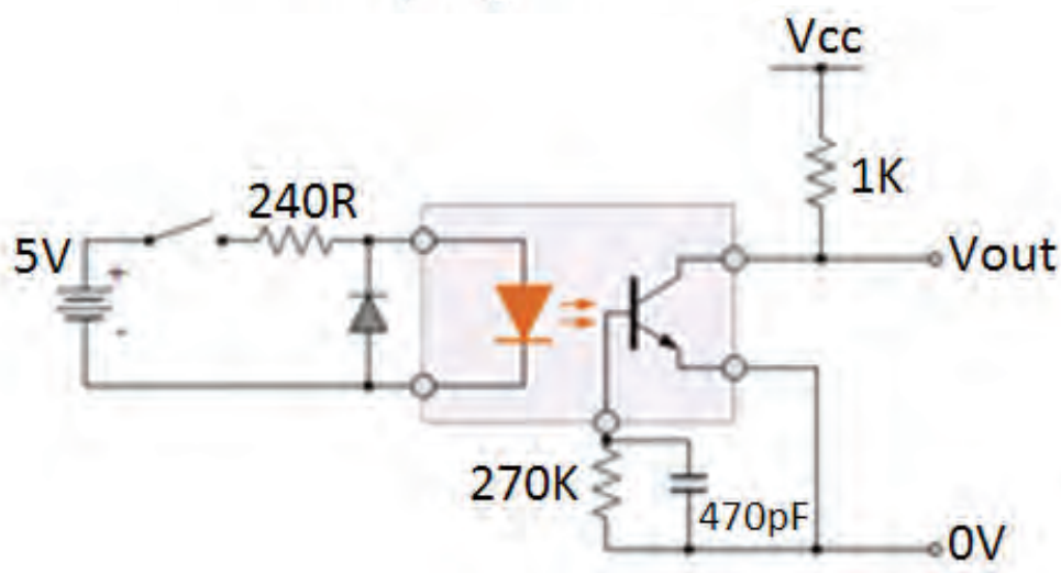
شکل ۲-۴۳- یک نمونه سنسور زیر کارتريج و مدار الکترونیکی آن
