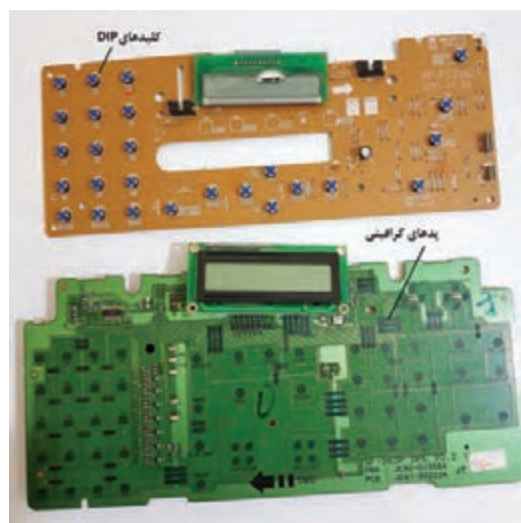
شکل ۳-۴۱- دونه پنل دستگاه چهارکاره
