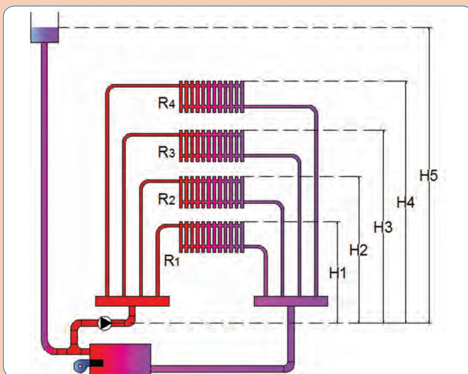
شکل ۴- تحلیل مؤلفه های معادله برنولی در سیستم گرمایش
