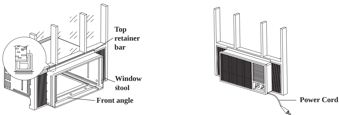
شکل ۹- نصب کولر
