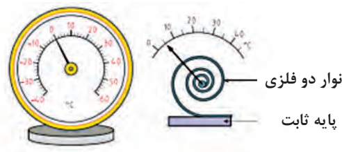
شکل ۱۰- دماسنج دوفلزی حلزونی شکل
