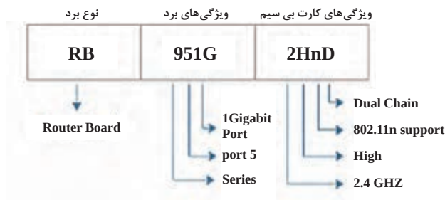
شکل ۵- نام‌گذاری مسیریاب
