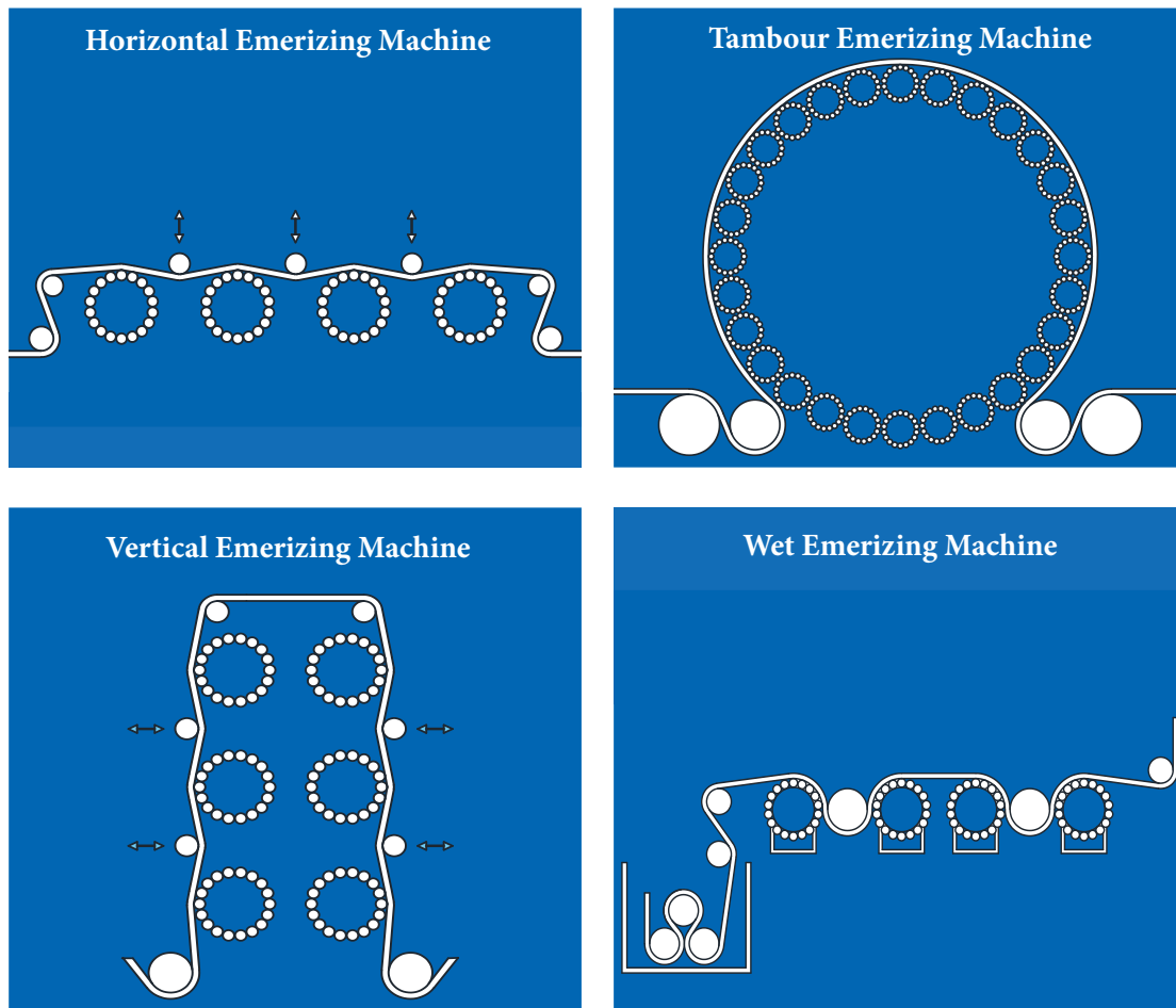
شکل ۱۲- انواع دیاگرام مسیر حرکت پارچه در ماشین سنباذه‌زنی
