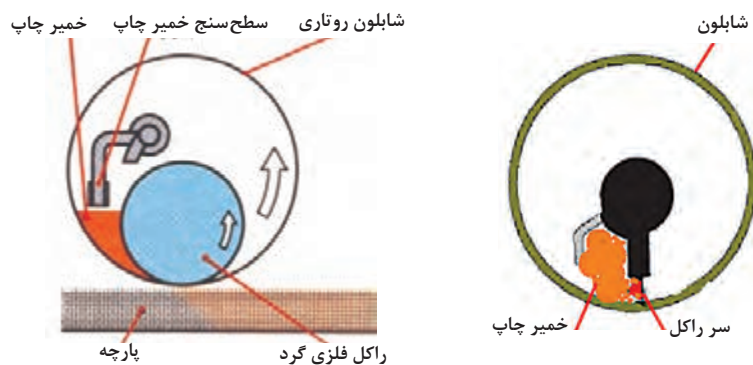
شکل ۲۰- راکل ثابت و راکل فلزی چرخان در چاپ روتاری
