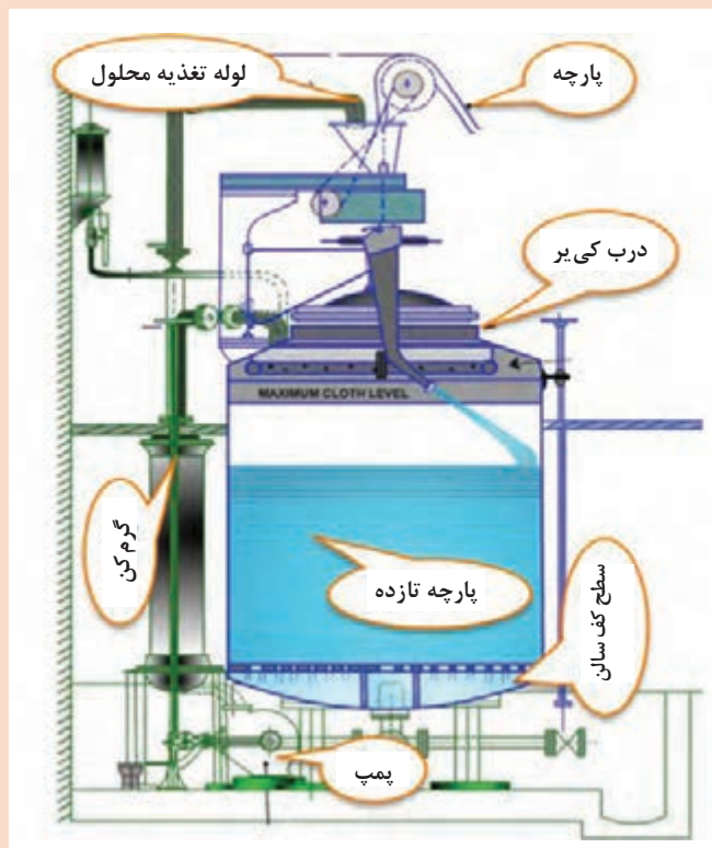
شکل ۶- نمایی شماتیک از ماشین کی‌یر (Kier) تحت فشار
