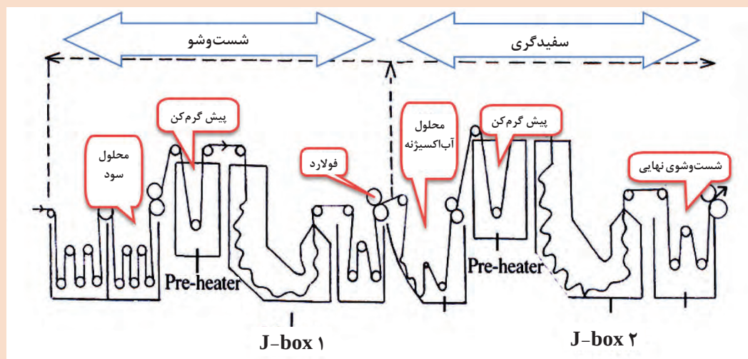
شکل ۹- مراحل پخت و سفیدگری هم زمان پارچه سلولزی
