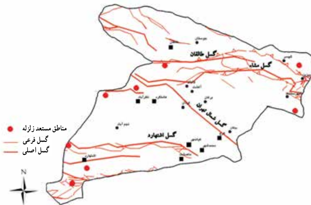
شکل ۱-۵- نقشه پراکنده گسل‌های اصلی استان
