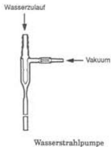
۲۰-۳- پمپ خلاء
