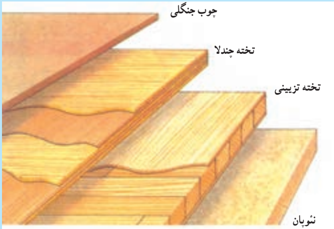
مقاطع‌ی از تخته‌های نئوپان، چندلای، چوب جنگلی و تخته‌های تزیینی
