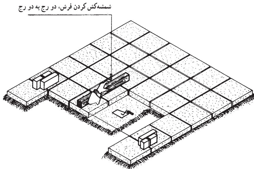
شکل ۹-۱۳- دو رج به دو رج فرش موزاییک
