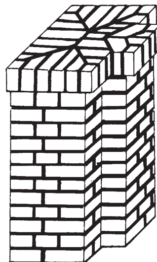
شکل ۳۳-۲- پرسپکتیو یا نمای هره‌چینی
