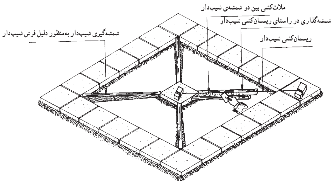
شکل ۹-۲۱- شمشه گیری شیب‌دار به وسیله کرم‌ها
