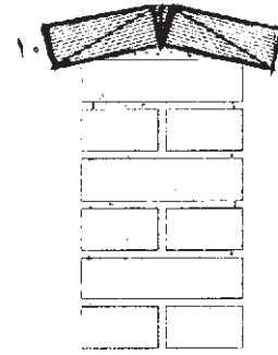
شکل ۲-۲۲ - هره چینی شیب دار انتهای
