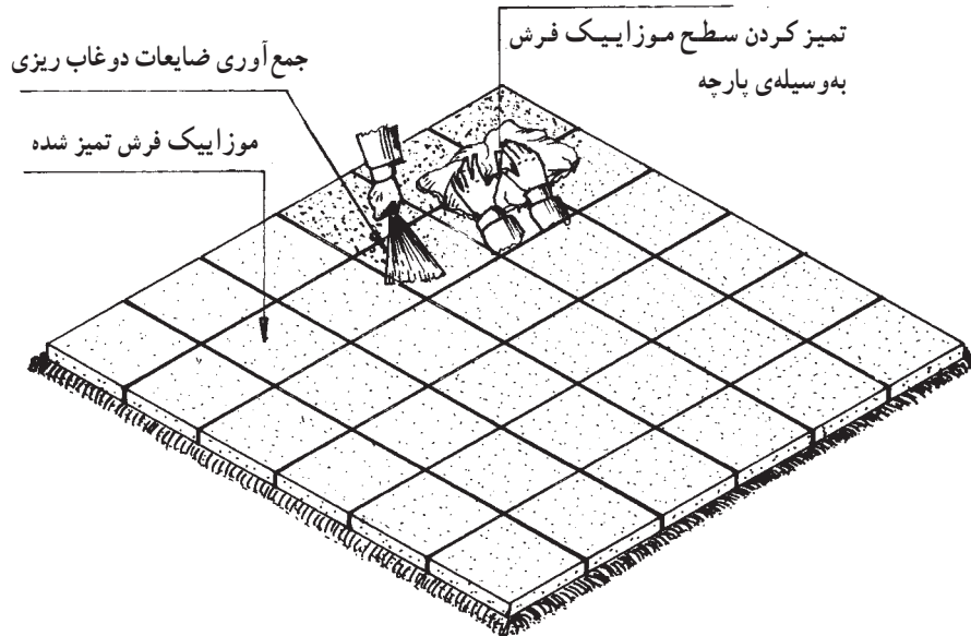
شکل ۱۴-۹- نحوه‌ی تمیز کردن سطح موزاییک فرش
