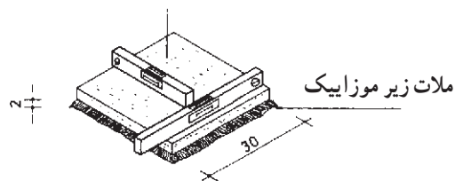
ترازسازی کرم موزاییک به شکل چپ و راست
