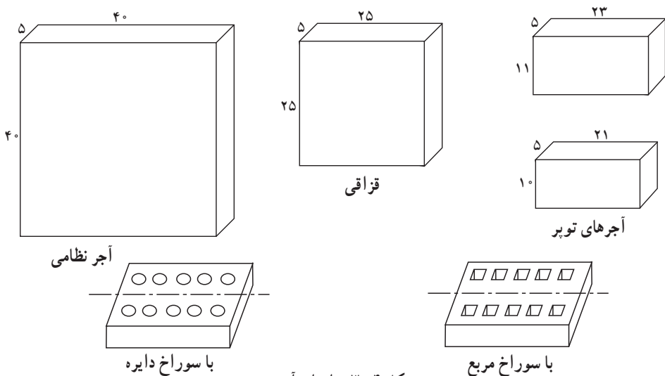
شکل ۳-۴-۵ انواع آجر
