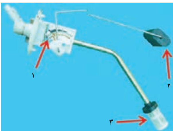
شکل ۱۴-۱- سوخت‌نمای دیجیتالی
