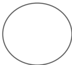
شکل ۲۴-۶ رسم مسیر
