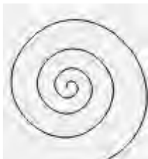
شکل ۷-۱۰ مارپیچ گسترشی
