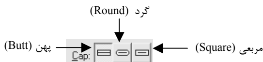
شکل ۸-۸۵ تنظیمات Cap
