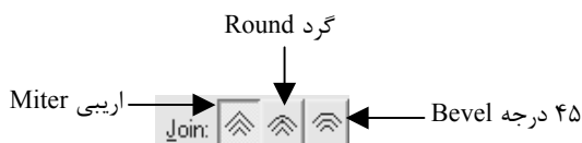
شکل ۸-۸۶ تنظیمات Join
