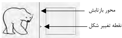
شکل ۶۰-۴ محور بازتابش
