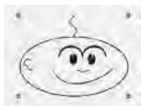
شکل ۴-۴۱ انتخاب شکل
