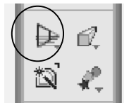
شکل ۲۰-۱ ابزار پرسپکتیو
