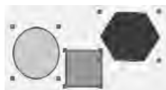
شکل ۶-۵۸ انتخاب اشکال
