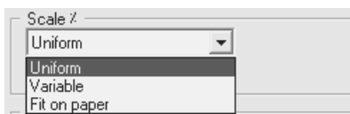
شکل ۹-۱۸ بخش Scale %
