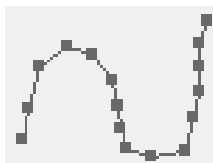
شکل ۱۸-۸ انتخاب مسیر
