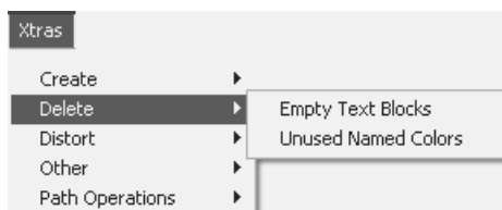
شکل ۸۱-۸ منوی Delete
