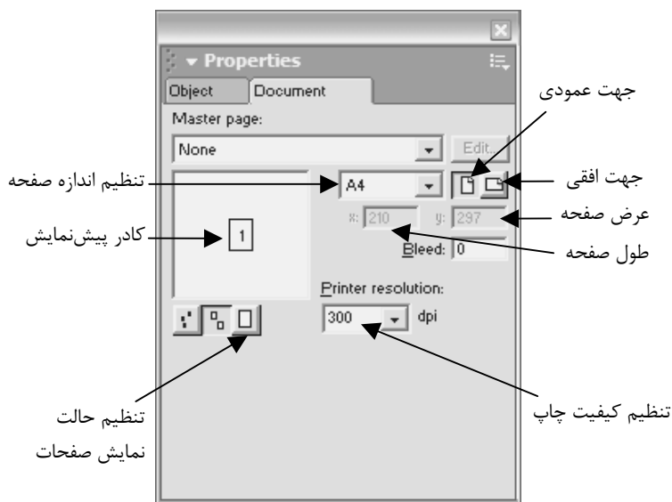
شکل ۱-۶ پنل Document
