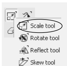
شکل ۴-۴۹ ابزار Scale
