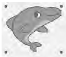
شکل ۴-۵۰ انتخاب شکل
