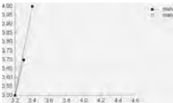
شکل ۶۹-۷ نمودار Scatter داده‌های شکل ۶۳-۷
