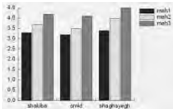
شکل ۷-۶۴ نمودار میله‌ای داده‌های شکل ۷-۶۳
