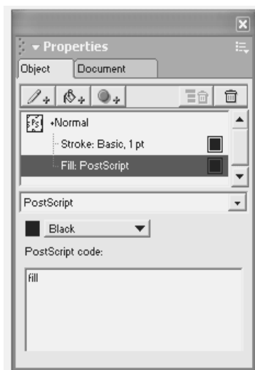
شکل ۴۵-۵ گزینه PostScript
