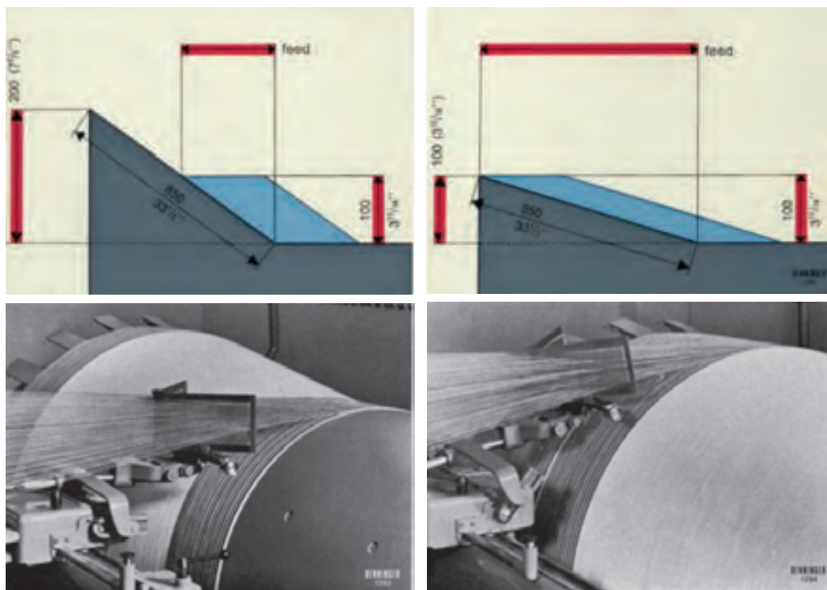
شکل ۴-۲- ساپورت ماشین چله‌پیچ بخشی
