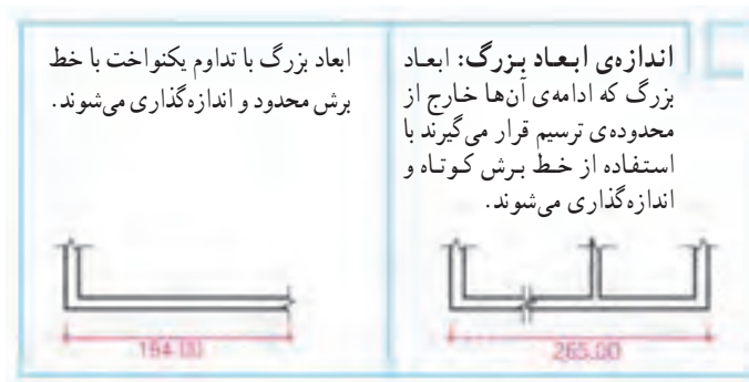
شکل ۱۵-۴- روش‌های اندازه‌گذاری
