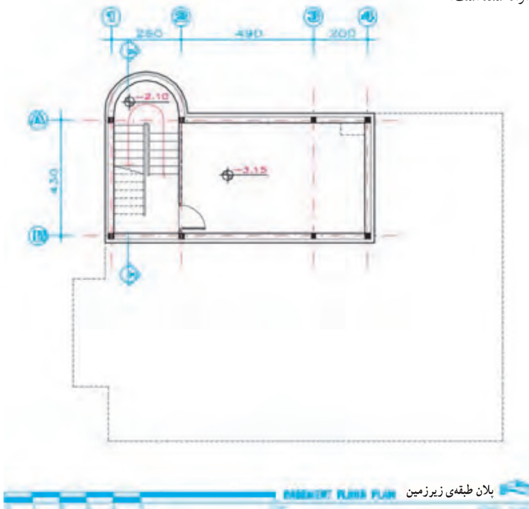
شکل ۴-۱۹- پلان زیرزمینی
