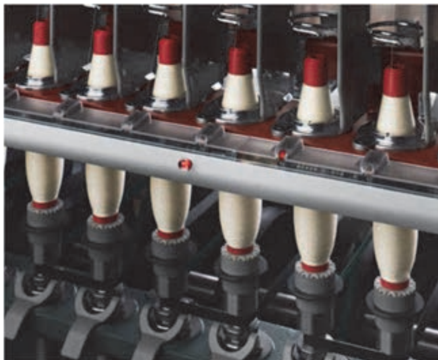
شکل ۳-۵ فاصله دو دوک متوالی در دستگاه رینگ
