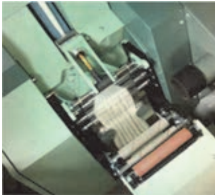
شکل ۳-۳۹ قسمت کشش در ماشین شانه
