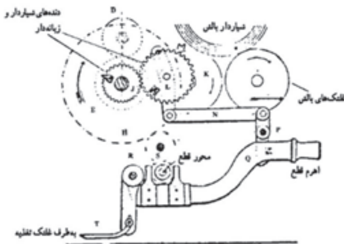
شکل ۳۲-۱ نمایی از مکانیزم قطع کن در دستگاه متکاپیچی
