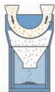
شکل ب ۱۶-۱ تمیز کننده بدون زننده
