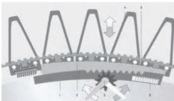
۲-۳۵ سیستم تنظیم فاصله کلاهدک و سیلندر PFS
