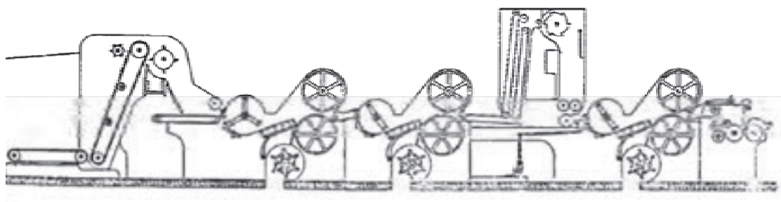
شکل ۱-۲۶ ماشین بالش با سه زنده و دستگاه تغذیه
