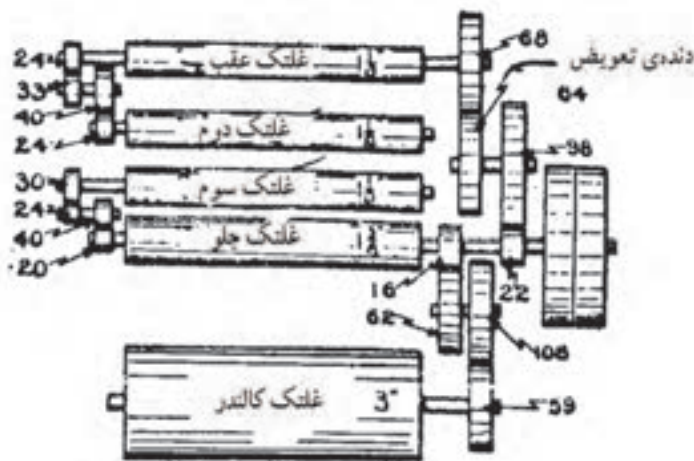
شکل ۱۶-۳: دیاگرام انتقال حرکت در قسمت کشش یک ماشین فتیله
