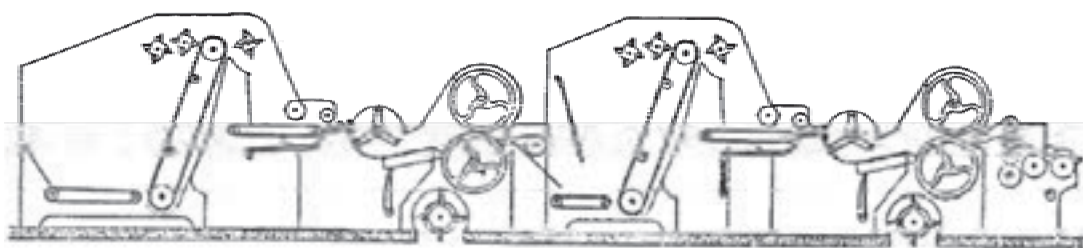
شکل ۱-۲۵ ماشین بالش با دو زنده و دو دستگاه تغذیه
