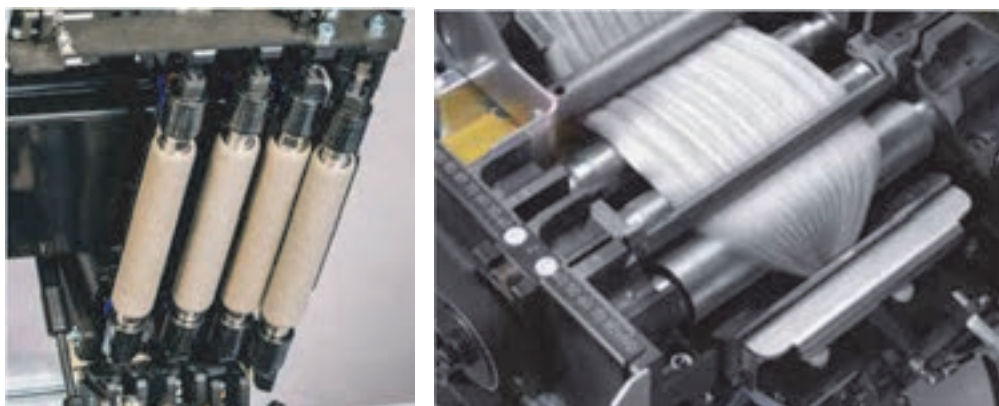
شکل ۳-۷-نمایی از غلتک های زیری کشش و غلتک های رویی در یک ماشین چند لاکنی
