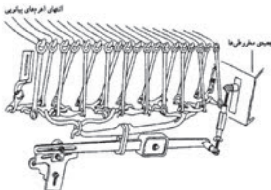
شکل ۲۲-۱: نمایشی از طرز اتصال اهرم‌های پیانویی
