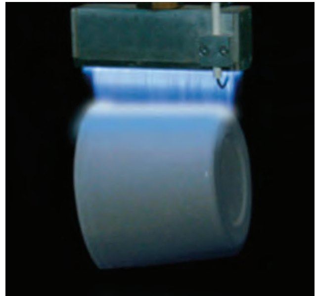
شکل های ۴۵-۳ روش شعله زنی
