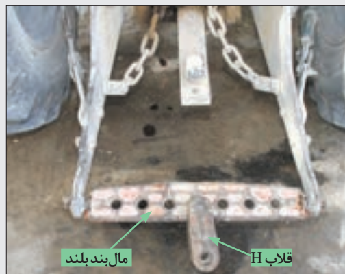
شکل ۱۵-۵- مال‌بند بلند برای اتصال ماشین هموارکننده نیمه‌سوار
