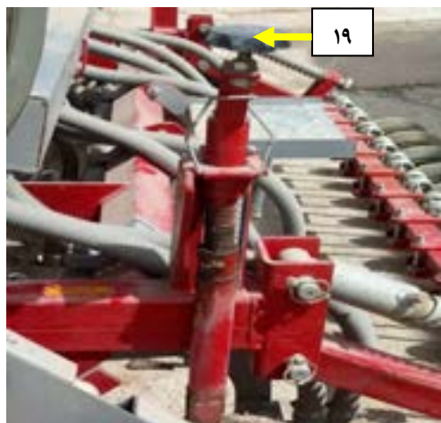
شکل ۳۹- اهرم تنظیم عمق کاشت
