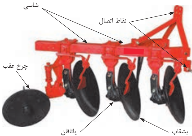
شکل ۸-۱. گاوآهن بشقابی
