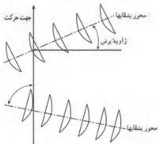
شکل ۱۷-۲. زاویه برش
