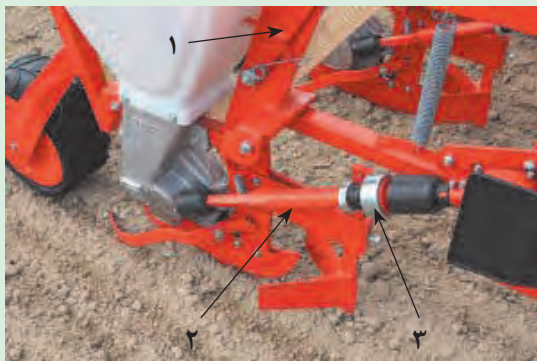
شکل ۲۷-۳. حذف واحد کارنده در یک نمونه ردیف‌کار
