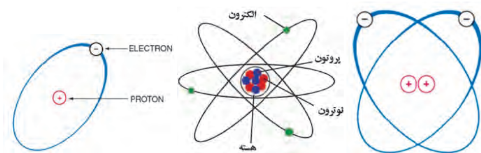
ساختمان اتم
