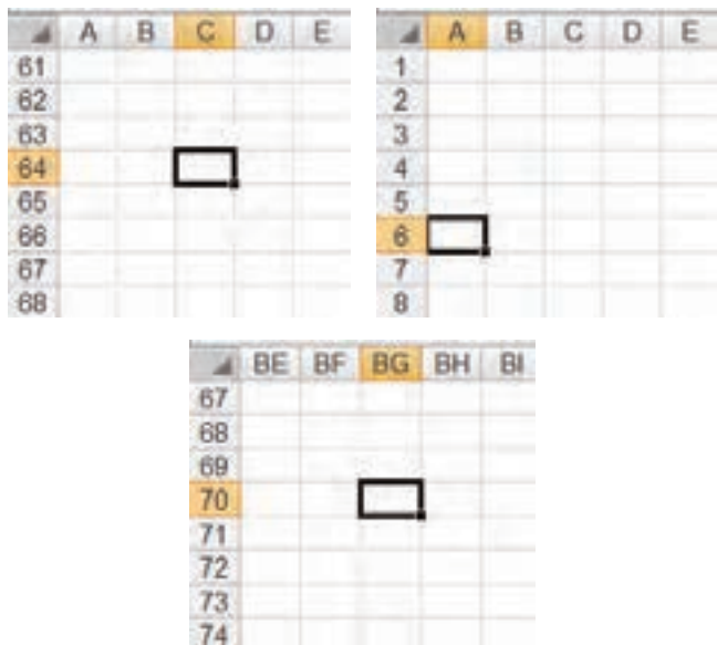
شکل ۱-۱۰ سلول‌های نمونه
