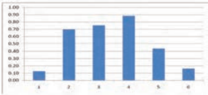
نمودار میله‌ای
