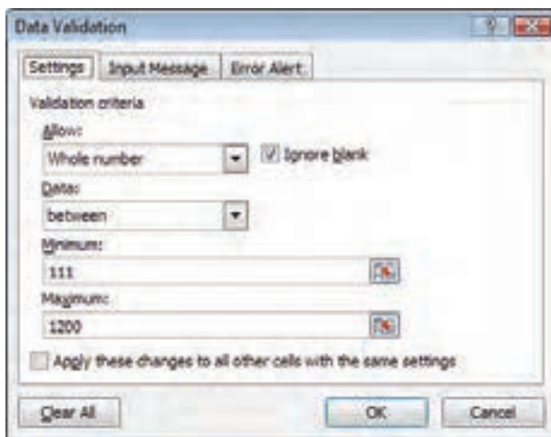
شکل ۸-۱۸ قید نمونه
