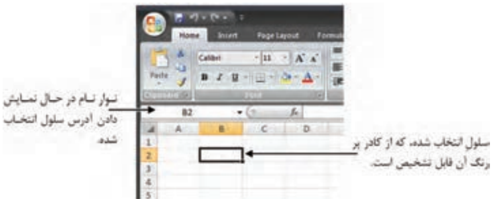
شکل ۱-۱۳ نوار نام
