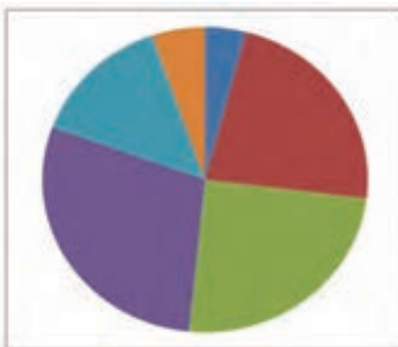
شکل ۱-۷ انواع نمودار
