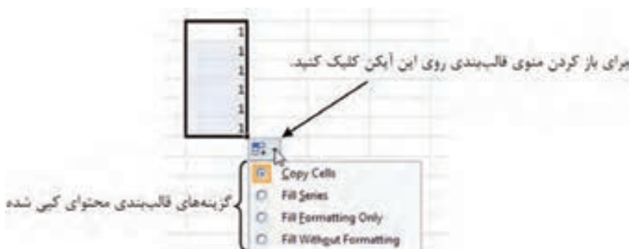
شکل ۳۱-۶ انتخاب‌های کپی
