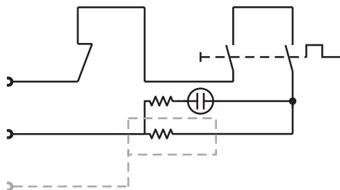
شکل ۷۳ نقشه ی مدار الکتریکی کتری برقی قسمتی از چای ساز
