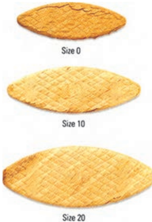
شکل ۸۱-۲ اندازه های اتصال بیسکوییتی
