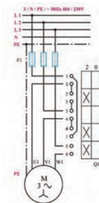
شمای حقیقی استاندارد IEC
