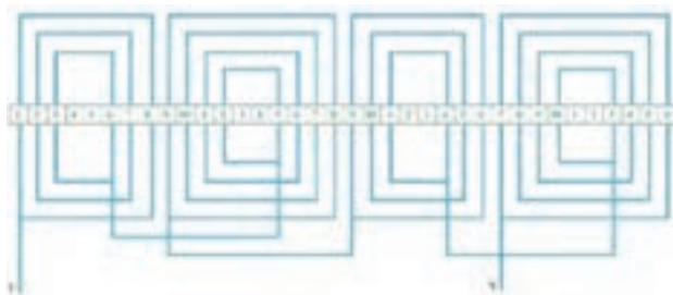
دیاگرام گسترده موتور یک فاز با ۴ قطب و ۲۴ شیار
