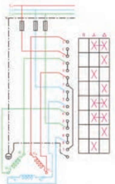
شمای حقیقی کلید راه اندازی ستاره - مثلث
