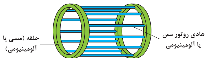
شکل ۵ - روتور قفسی
