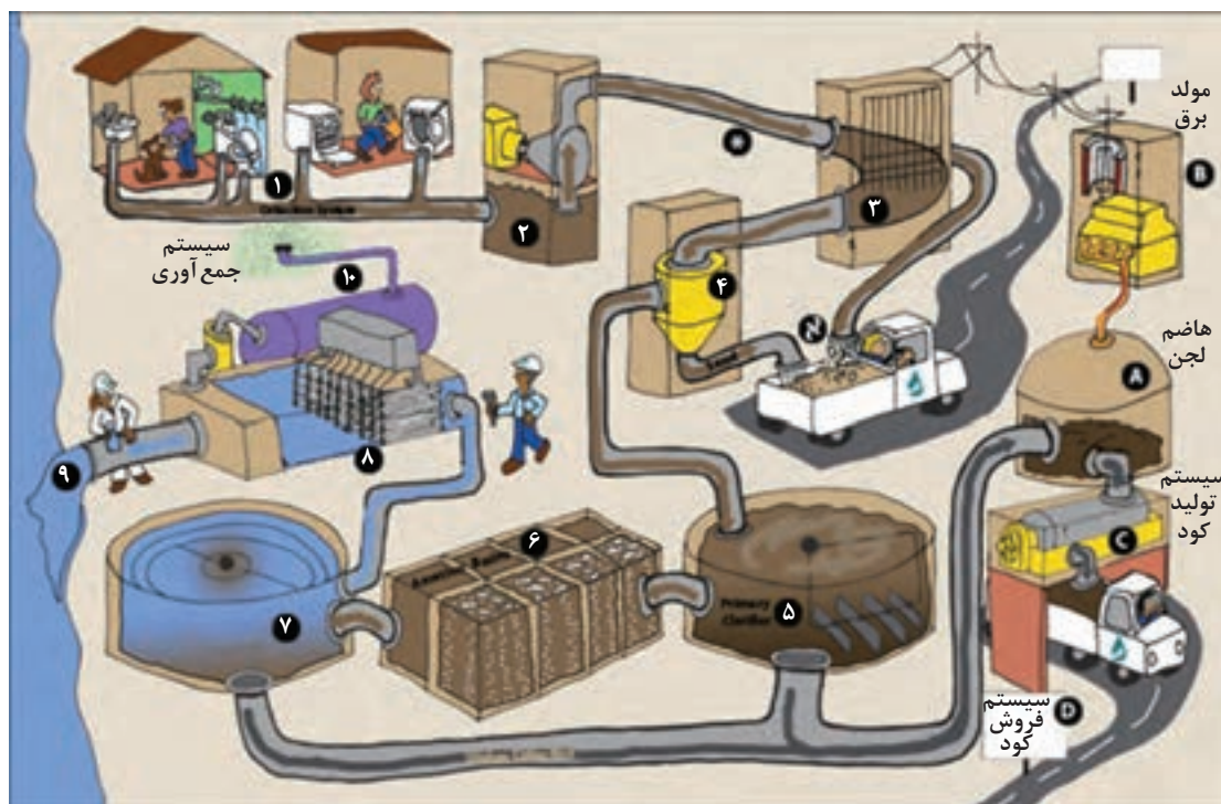
شکل ۱- تولید فاضلاب و استفاده مجدد پساب در اجتماع ۱- سیستم جمع آوری فاضلاب ۲- پمپاژ فاضلاب ۳- آشغال گیر ۴- دانه گیر ۵- زلال ساز اولیه ۶- حوضچه هوادهی ۷- زلال ساز ثانویه ۸- کلر زنی ۹- تخلیه فاضلاب تصفیه شده ۱۰- استفاده مجدد در کشاورزی
