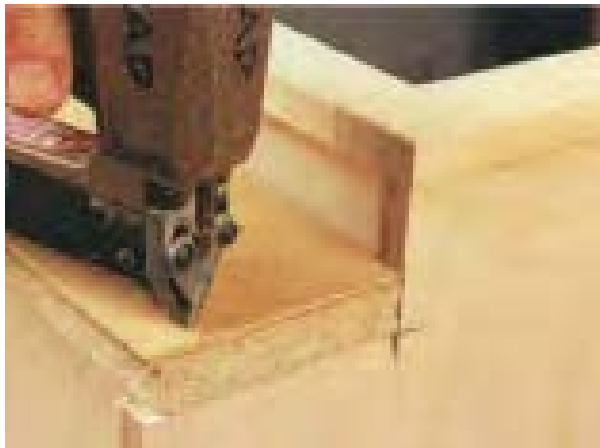
شکل ۲۱-۸- اتصال سه‌لایی به تخته خرده چوب.
