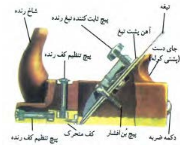
شکل ۲-۲- رنده‌ی دو تیغه چوبی.
