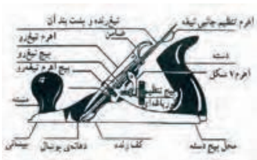
شکل ۲-۳- رنده‌ی دو تیغه فلزی
