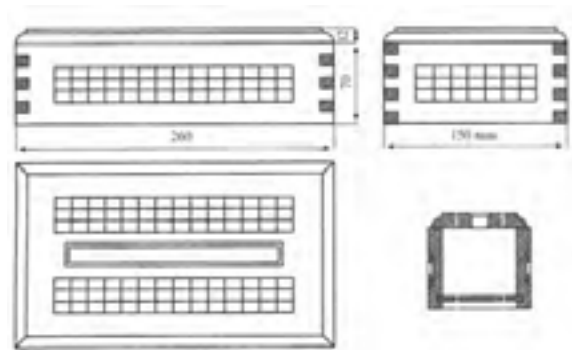
شکل ۹-۷۳ - نقشه‌ی سه‌نمای معبوی دستمال کاغذی به همراه برش عرضی.
