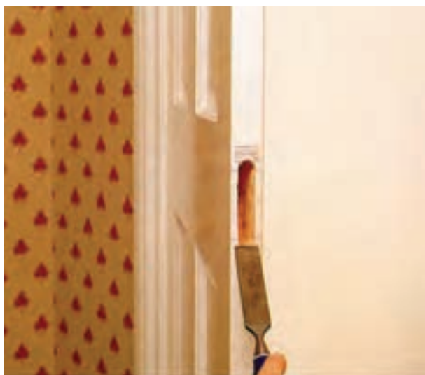
شکل ۱۰-۴۶-۱- درآوردن ممل کامل قفل.
