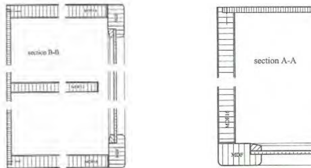
شکل ۱۲-۸۳. نماها و برش‌های جمعیه کمک‌های اولیه چوبی.
