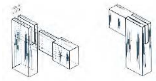
شکل ۱۱-۱۴- فاق و زبانه.
