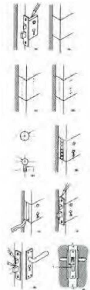
شکل ۱۱-۵۲- مراحل مختلف جاسازی قفل.
