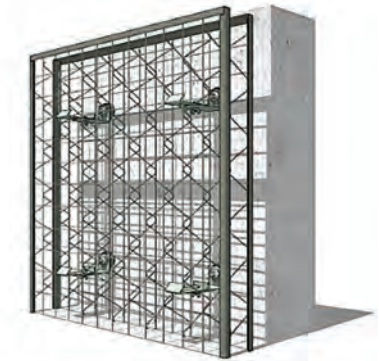
پانل فلزی در سیستم شبکه‌ای داربستی
