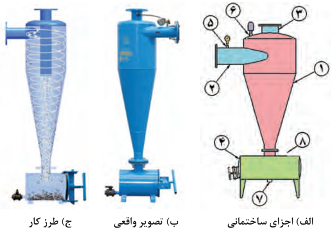
شکل ۲۱- هیدروسیکلون
