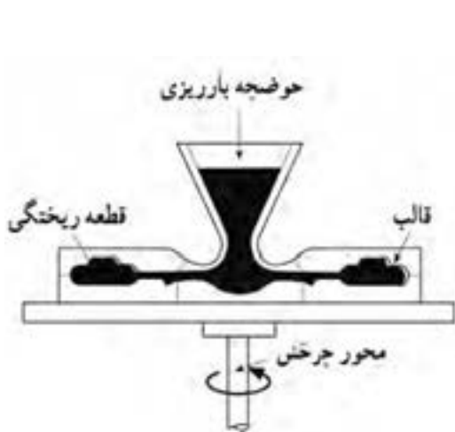
شکل ۳۳-۳- روش ریخته‌گری چرخشی گریز از مرکز
