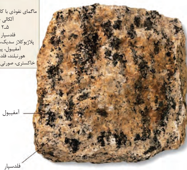
شکل ۲-۲۹- سینیت
