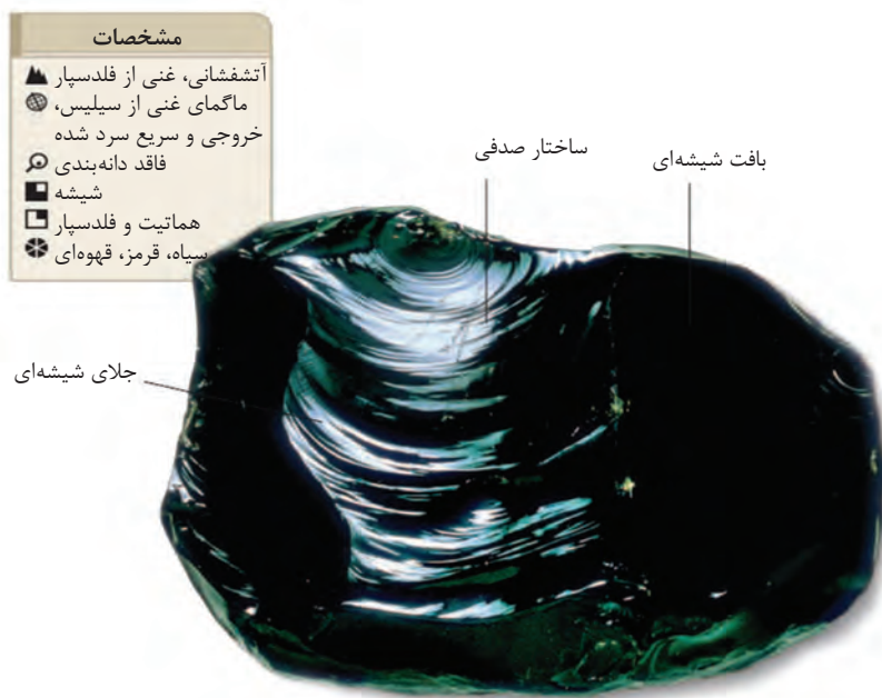
شکل ۲-۲۶- ابسیدین
