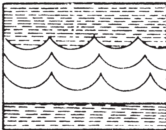
شکل ۲-۴۰- ریپل مارک (۴)
