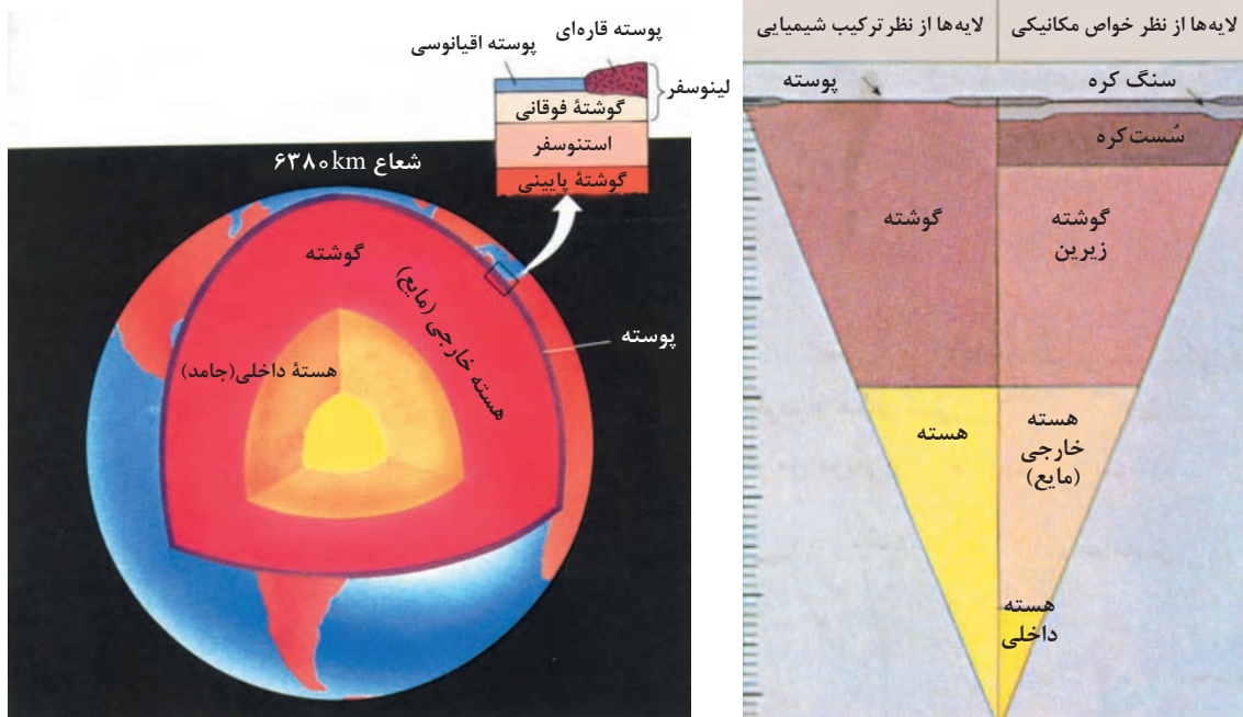
شکل ۲-۶- لایه‌های زمین (۴)
