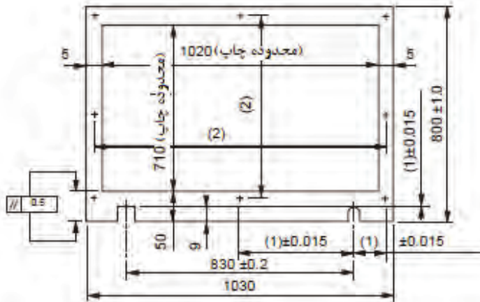
شکل ۷۴- ابعاد پلیت
