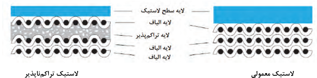
شکل ۵۶- انواع لاستیک
