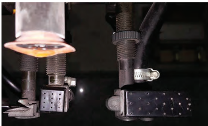
شکل ۱۶- دمنده‌های پشت
