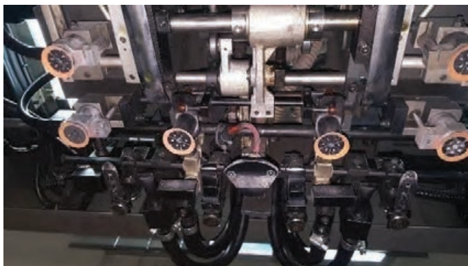
شکل ۱۲- مکنده‌های آپارات
