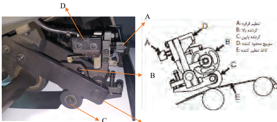
شکل ۲۴- دو تا بگير مکانیکی
