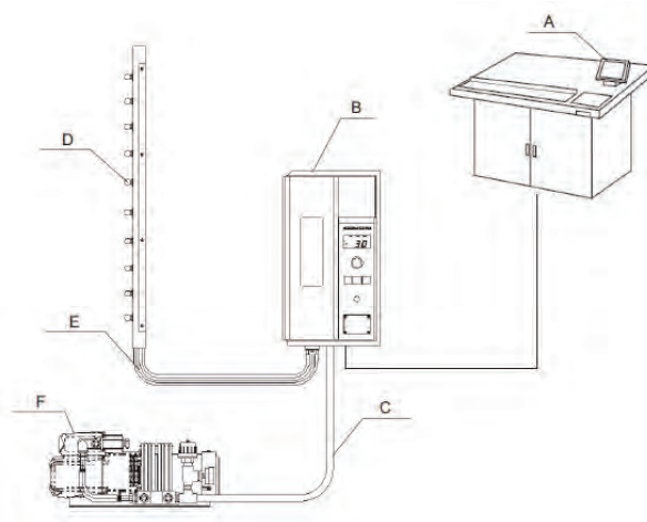
شکل ۵۴- سیستم پودرپاش
