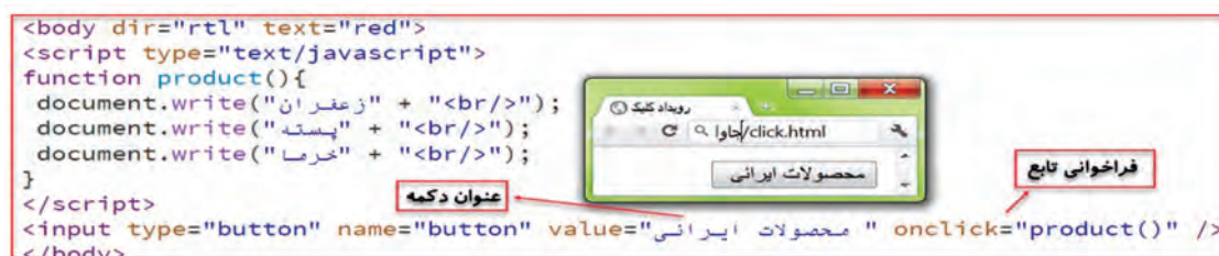
شکل ۶- رویداد onclick
