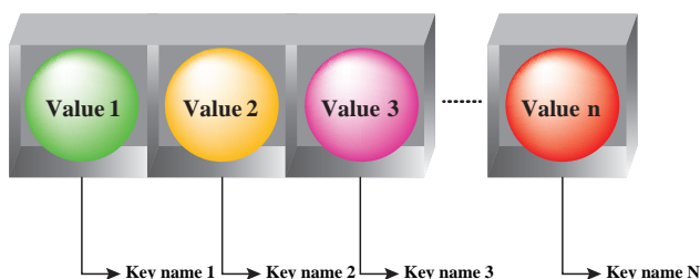
شکل ۱۳- آرایه انجمنی
