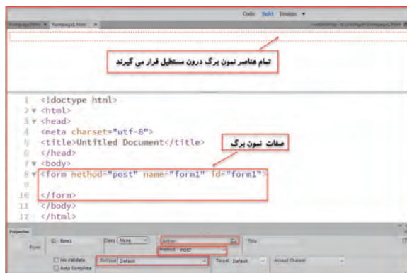
شکل ۴۵- نمایش برچسب نمون برگ
