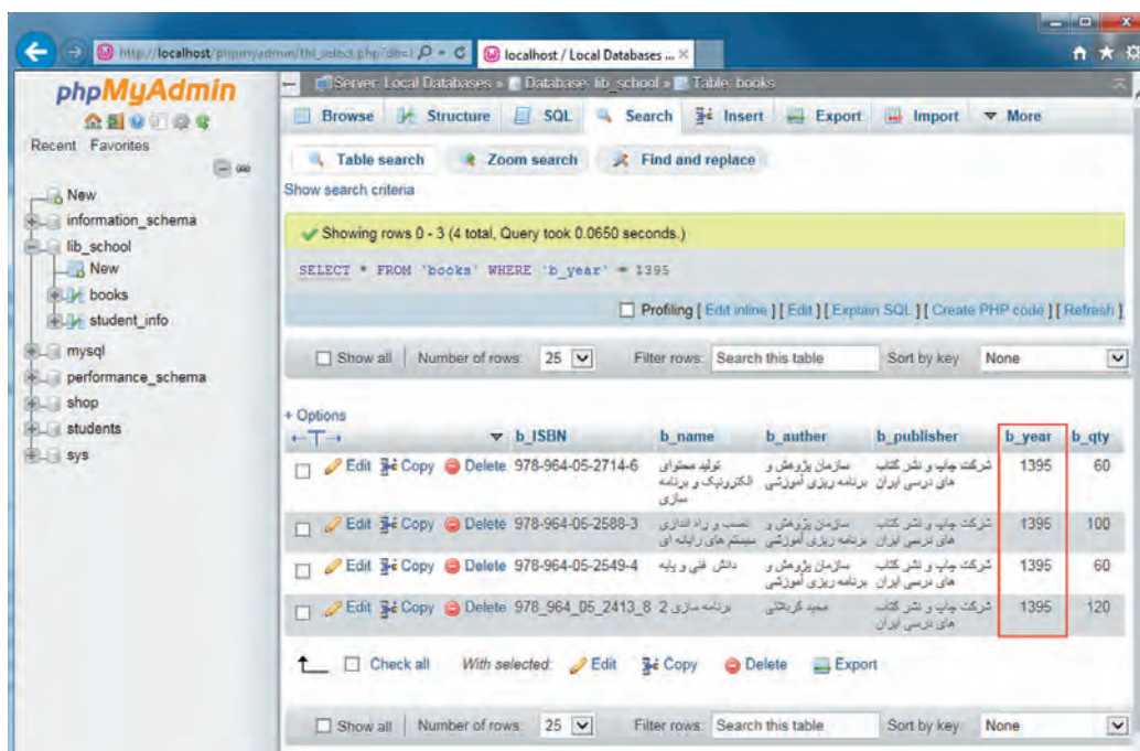
شکل ۳۵- نتیجه پرس‌وجو پس از اعمال محدودیت
