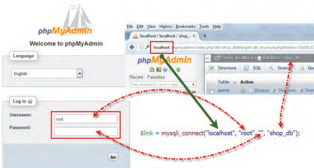
شکل ۴۵- معادل دستور mysqli_connect در phpMyAdmin
