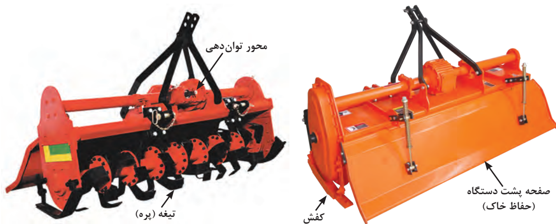
شکل ۱۴-۳- گاواهن دوار
