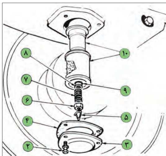
شکل ۳۳-۲- تعویض فیلتر هیدرولیک
