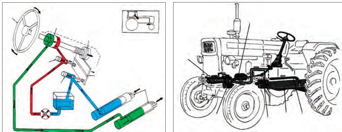
الف - سیستم فرمان نیمه هیدرولیک
