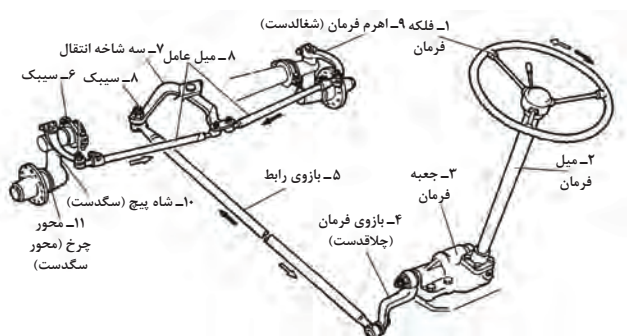
شکل ۳۶-۳- اجزای فرمان مکانیکی
