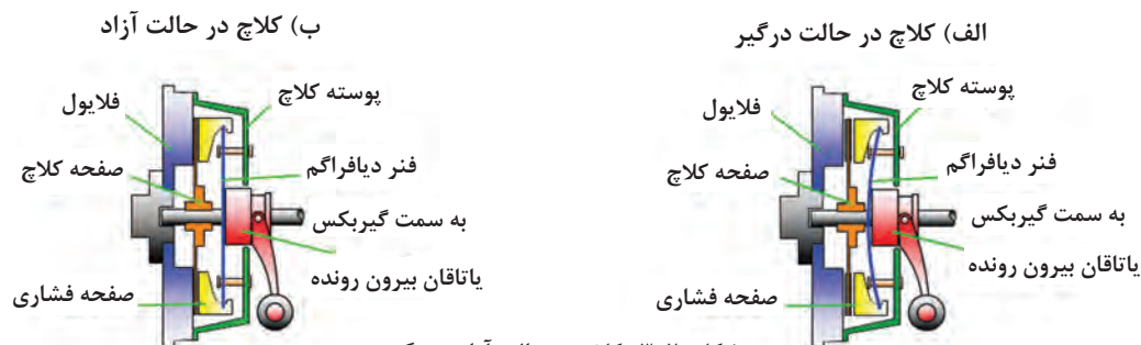
شکل ۳-۲۰- کلاچ در حالت آزاد و درگیر
