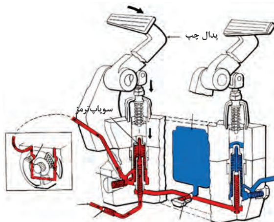
شکل ۳۸-۳- اجزای ترمز تراکتور
