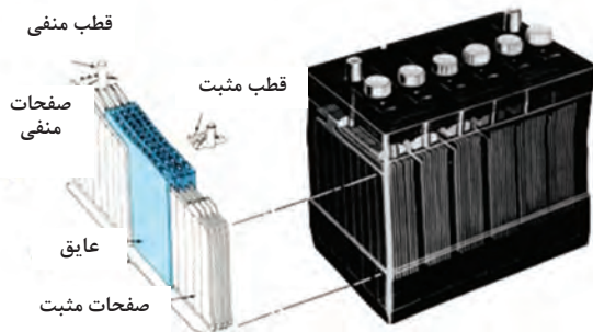
شکل ۷-۳- ساختمان باتری
