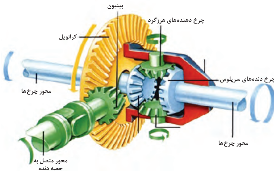
شکل ۲۲-۳- اجزای دیفرانسیل
