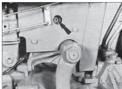
شکل ۳۹-۲- بازدید سطح روغن جعبه فرمان تراکتور ۲۸۵
