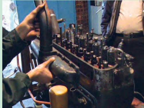
شکل ۴۳. باز کردن مانیفولد تراکتور U650
