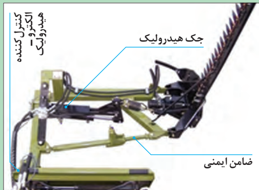
شکل ۱۷- دروگر شانه‌ای با سیستم محرک ارتعاشی
