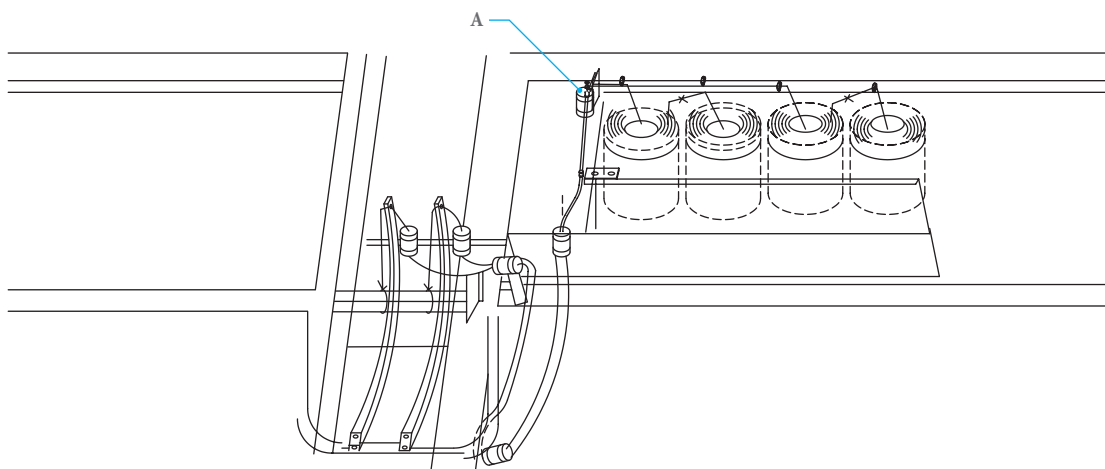
شکل ۸۸- نقشه راهنمای نخ کردن بسته‌بند مدل ۳۶۹ برچین کار
