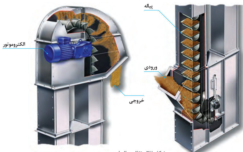
شکل ۲۷- نقاله پیاله‌ای
