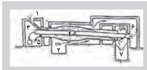
شکل ۲-۸- کوره دوار خفته: ۱- کلوخه سنگ گچ به کوره ریخته می‌شود ۲- آتسخانه ۳- گاز داغ به دور کوره گردنده دمیده می‌شود و از آن‌جا به درون کوره و سپس به دودکش می‌رود ۴- درون کوره ۵- مه بخار آب که از سنگ گچ برخاسته، مکیده می‌شود ۶- هوای تازه به کوره دمیده می‌شود ۷- کلوخه‌ی گچ پخته از کوره بیرون می‌ریزد
