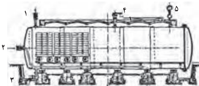
شکل ۱۲-۶- دستگاه پخت آجر ماسه آهکی: ۱- خروجی بخار آب ۲- ورودی بخار آب ۳- پس آب ۴- دریچه اطمینان ۵- فشارسنج
