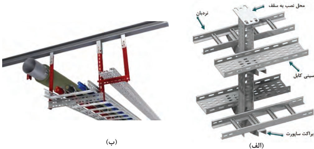
شکل ۵۹- ساپورت
