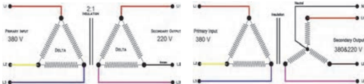
شکل ۱۸- تعیین خطوط برق شناور
