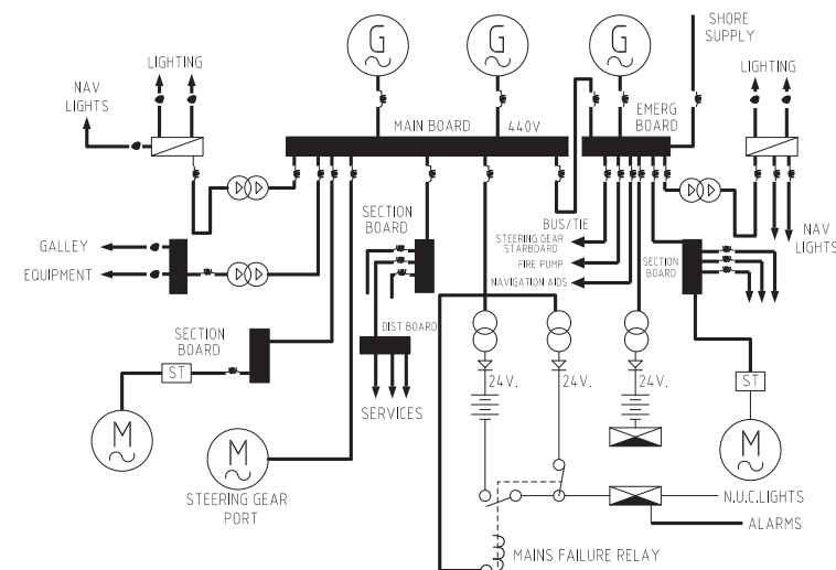
شکل ۱۷- سیستم توزیع جریان الکتریکی در شناور
