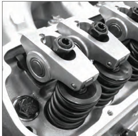
مجموعه اسبک های غلتکی در موتور OHV دارای تنظیم کننده هیدرولیکی ویاناقان رولبرینگ
