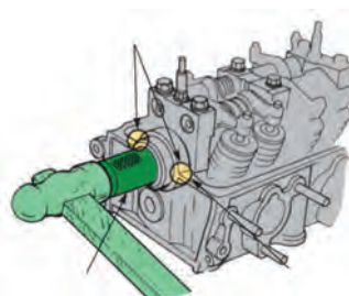
شکل ۱-۵۵ نحوه تعویض کاسه نمد میل سوپاپ با استفاده از ابزار مخصوص
