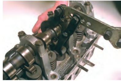
استفاده از فنر سوپاپ جمع کن اهرمی مخصوص در برخی از سرسیلندرها
