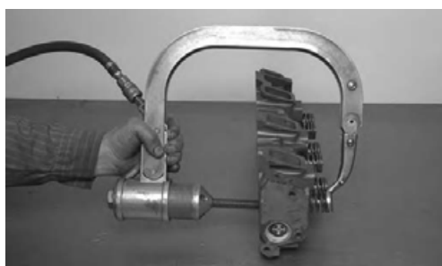
استفاده از فنر سوپاپ جمع کن پنوماتیکی
