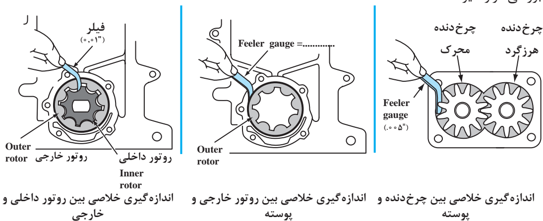
شکل ۲۸-۴ بررسی خوردگی و سایدگی اجزای داخلی پمپ
