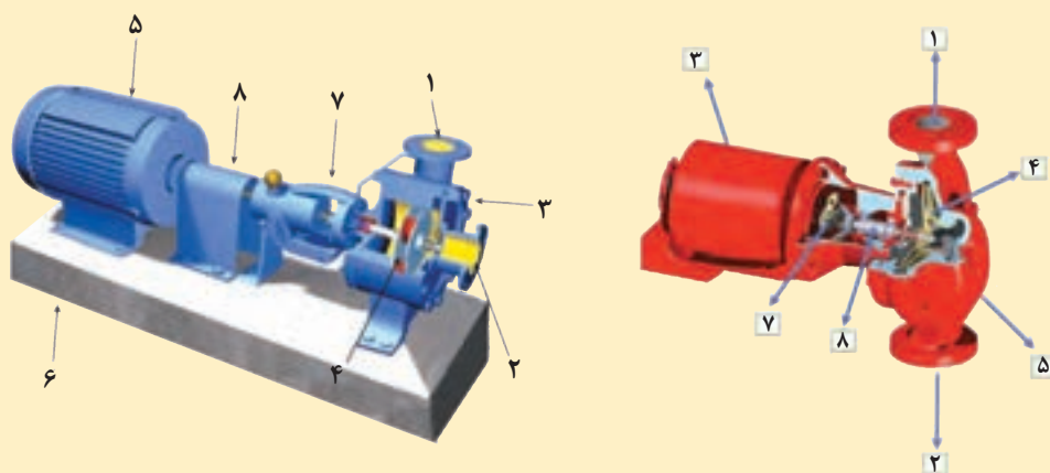
اجزای الکترو پمپ زمینی - اجزای الکترو پمپ خطی
