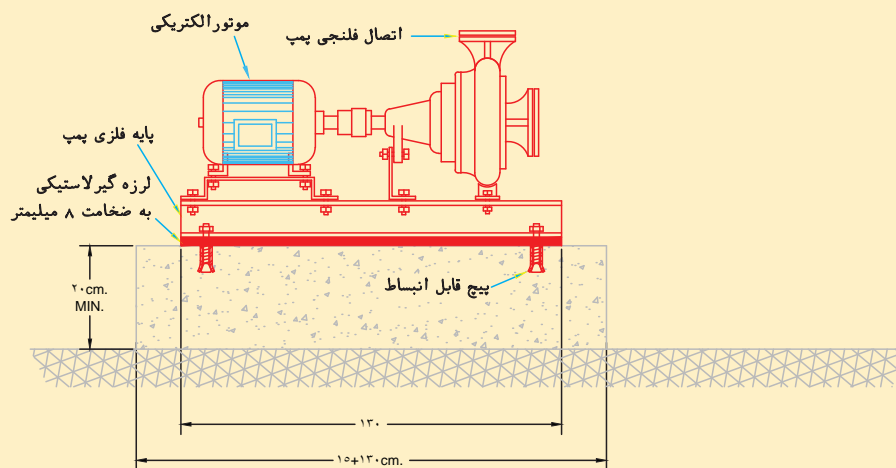
جزئیات نصب الکتروپمپ زمینی بر روی فنداسیون الف) پلان نمای از بالا ب) نمای جانبی
