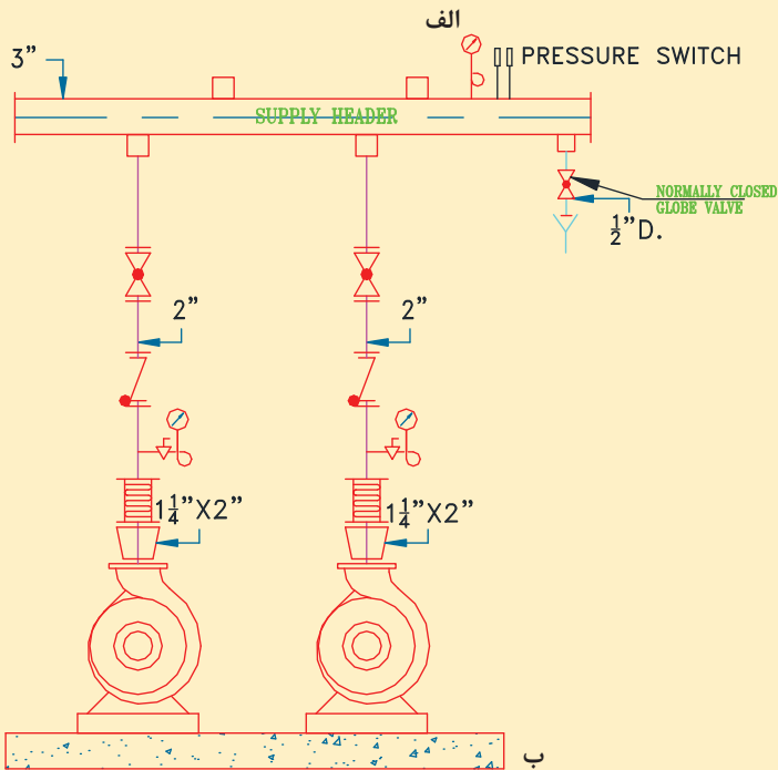
جزئیات نصب اجزای خط رانش پمپ زمینی به همراه کلکتور رفت الف) شماتیک نصب ب) نقشه لوله و اتصالات خط رانش
