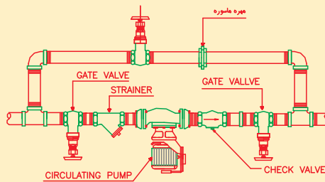
جزئیات نصب اجزای خط رفت و برگشت پمپ سیرکولاتور دیگ به مخزن آب گرم
