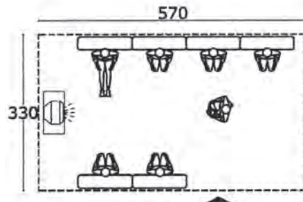
شکل ۱-۵۶- غذاخوردن بر روی زمین در نشیمن
