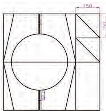
شکل ۳۸- خط‌کشی شکاف‌ها
