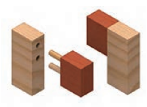
شکل ۲۶- اتصال دوبل
