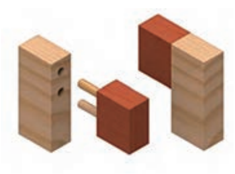
شکل ۲۶- اتصال دوبل
