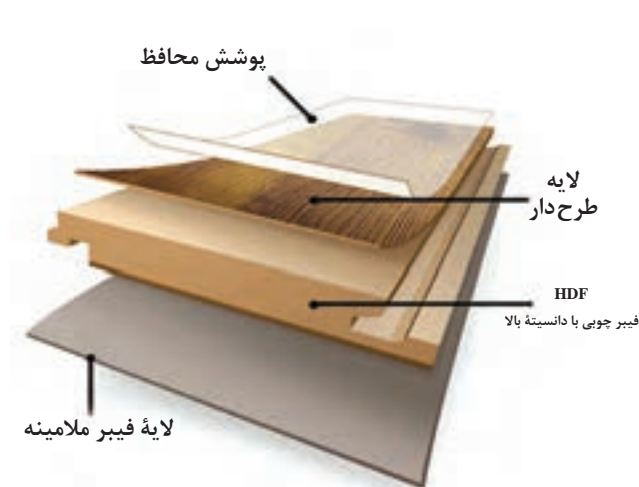
شکل ۱۲- انواع کف‌سازی باصفحات روکش‌دار
